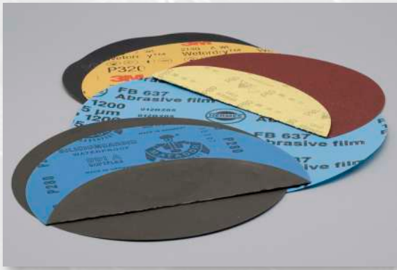
Disques à lapider de diverses marques autocollant / non-autocollant
